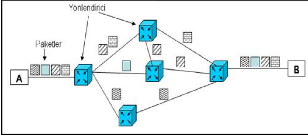
Şekil 2.2: Paket anahtarlama şebeke
