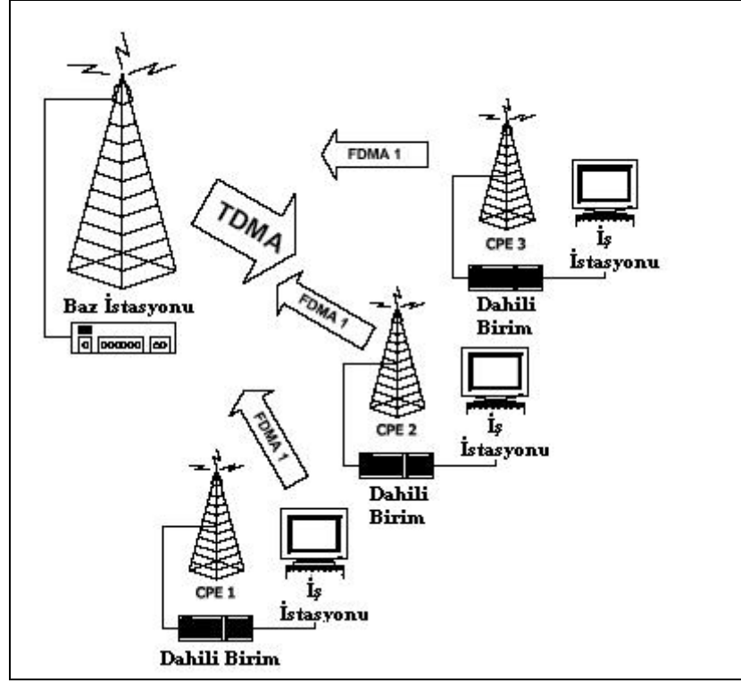
Şekil 2.11: LMDS’de veri alıŖta TDMA, veriŖte FDMA kullanımı
