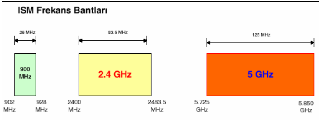
Şekil 1.4: ISM bant planı
