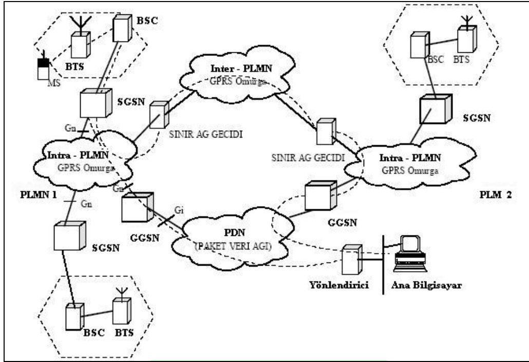
Şekil 2.9: GPRS sisteminde yönlendirme
