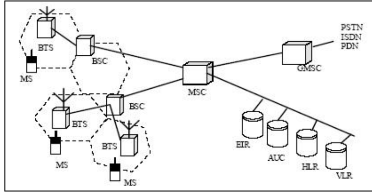
Şekil 2.5: GSM sistem yapısı
