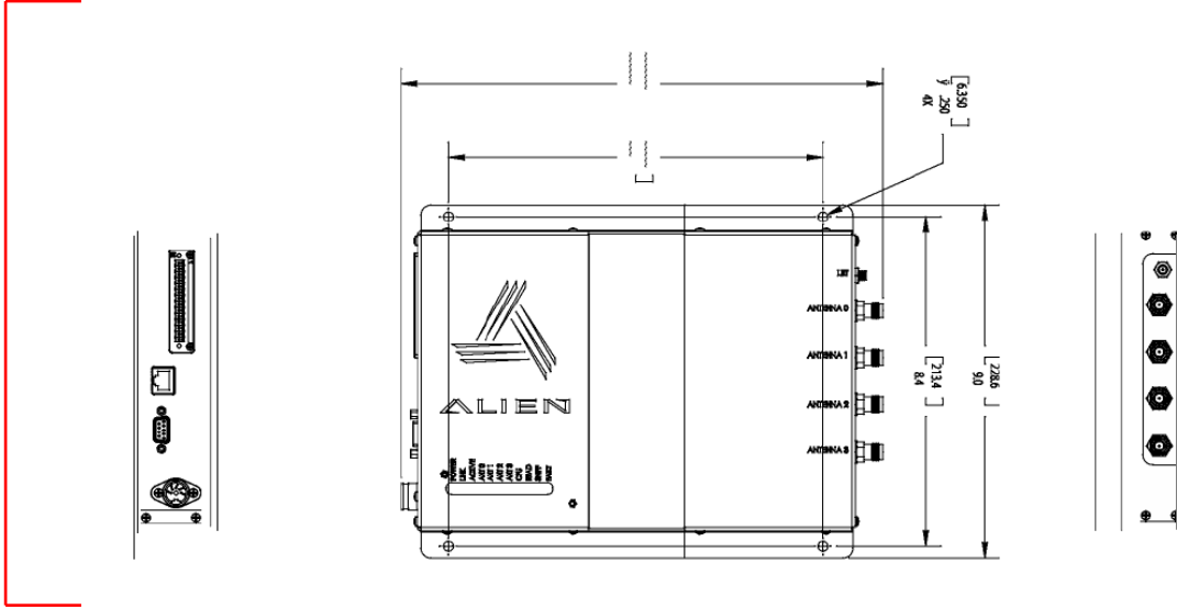
Şekil 6-4 Alien ALR-8800 RFID okuyucu Giriş/Çıkış bağlantıları ve genel görünüşü
