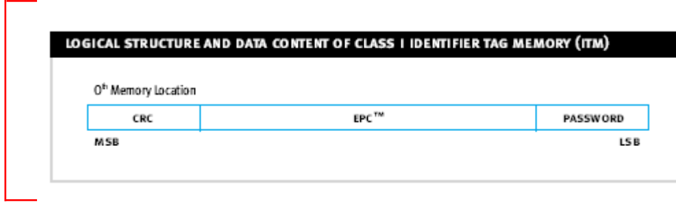
Şekil 5-2 Class I Kimlik Etiket Belleği (ITM) data içeriği ve organizasyonu
