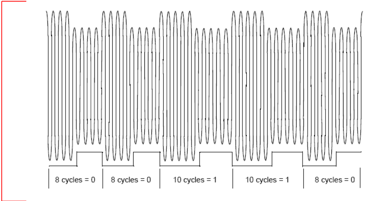
Şekil 3-3 FSK modülasyonlu sinyal F_c/8, F_c/10 . 3. PSK (Phase Shift Keying)
