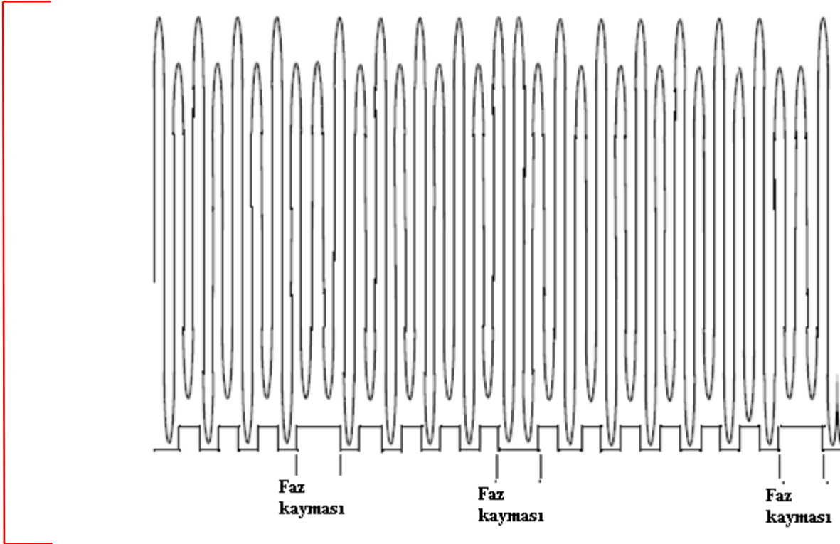
Şekil 3-4 PSK modülasyonlu sinyal
