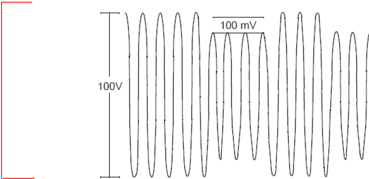
Şekil 3-1 Genlik modülasyonlu Backscatter modülasyonu
