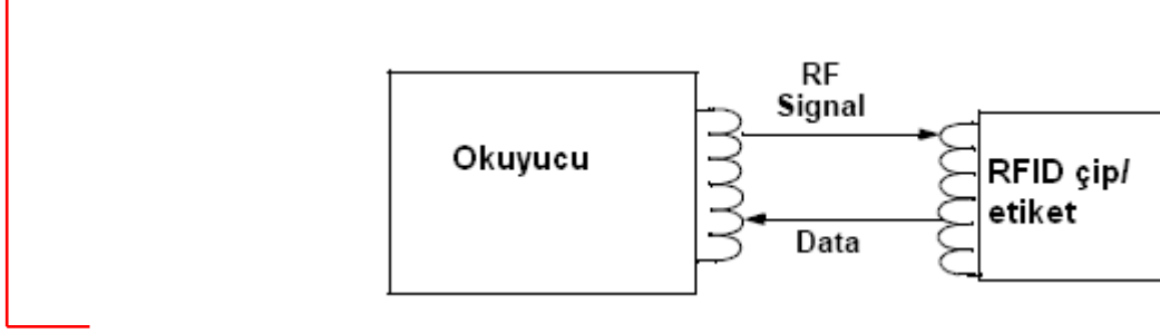
Şekil 3-5 Pasif RFID etiketin çalışma prensibi: okuyucudan gönderilen RF sinyali RFID çipinin bobininde indüklediği gerilim ile RFID çip enerjilenerek aynı anten üzerinden veri (data) bilgisini gönderir
